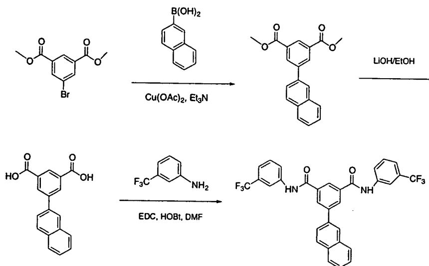
Scheme 1-E
